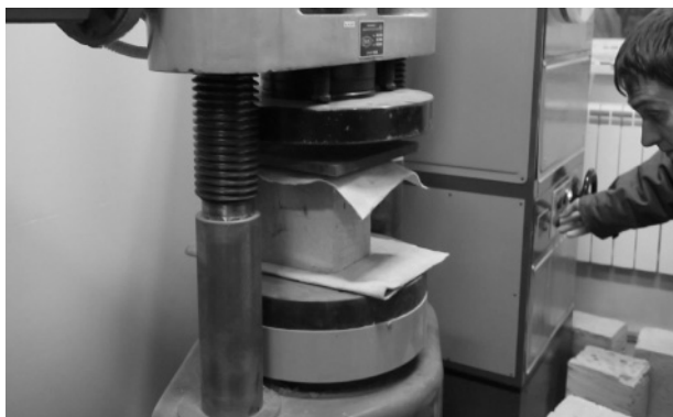
Рис. 1. Вигляд зразка перед випробуванням в дослідній машині Зим П-125
